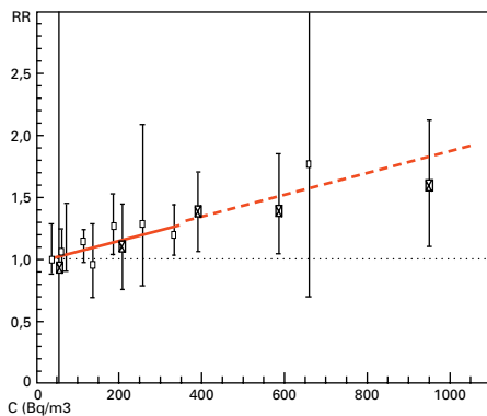
Relativní riziko plicní rakoviny (RR) vzhledem k průměrné koncentraci radonu v obydlich (C). Porovnání české studie (■) a zahraničních studií (□). Plná čára - model odvozený z 9 zahraničních studií přerušovaná čára - model RR = 1 + 0.087 C odvozený ze studie středočeský pluton.
